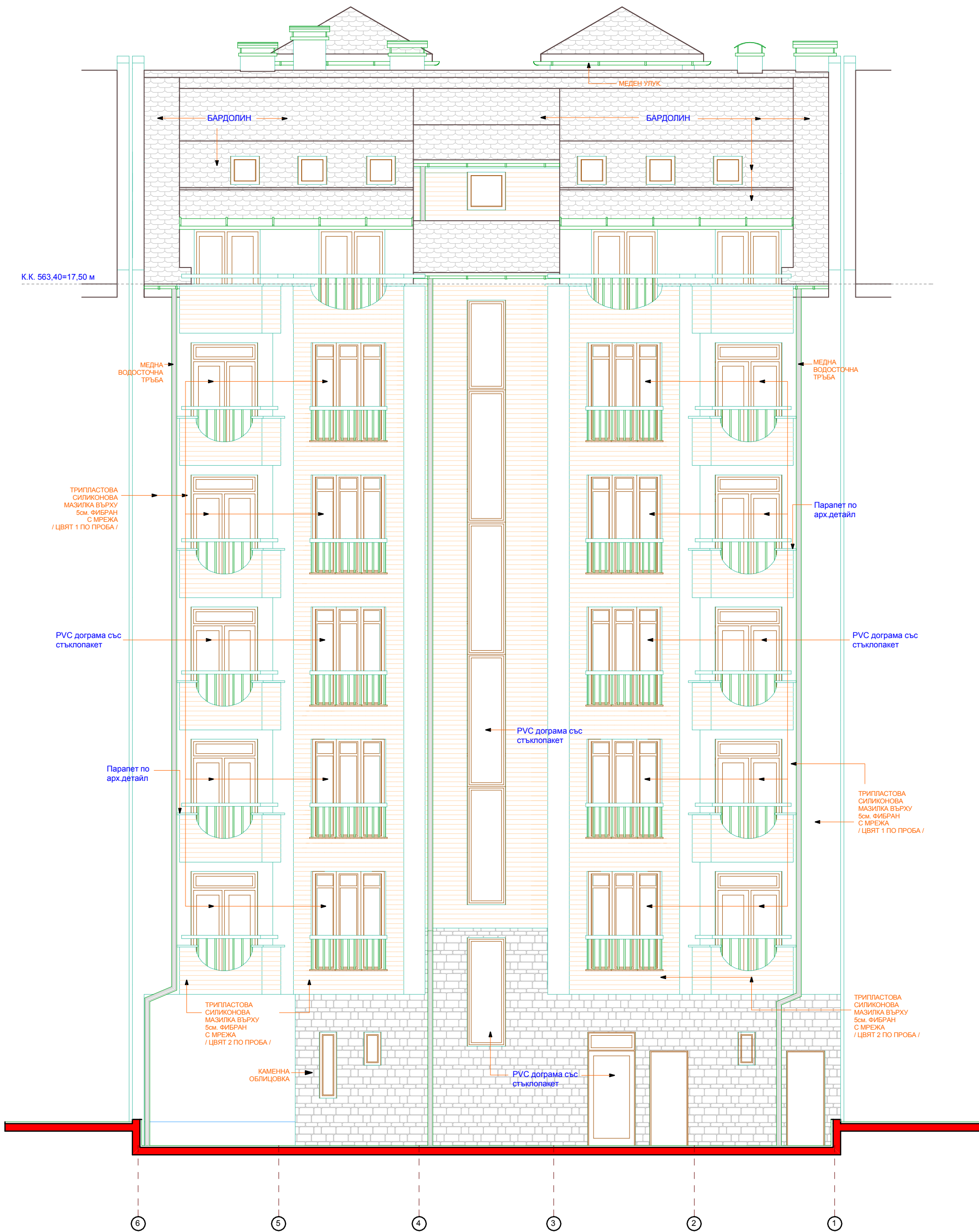
ФАСАДА ЗАПАД
