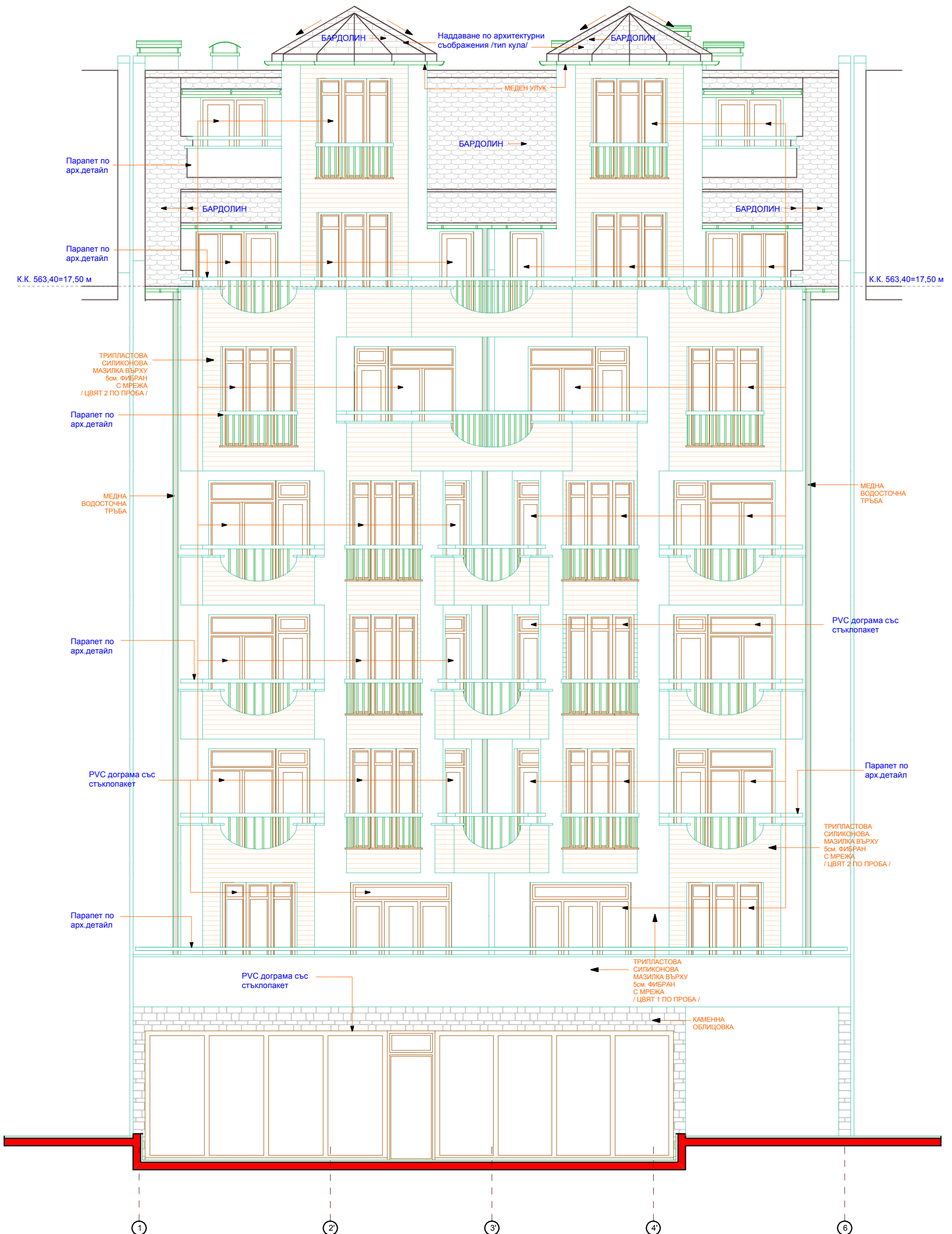
ФАСАДА ИЗТОК
