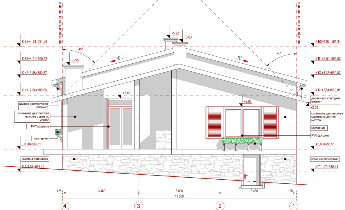
ФАСАДА СЕВЕР М 1:50
