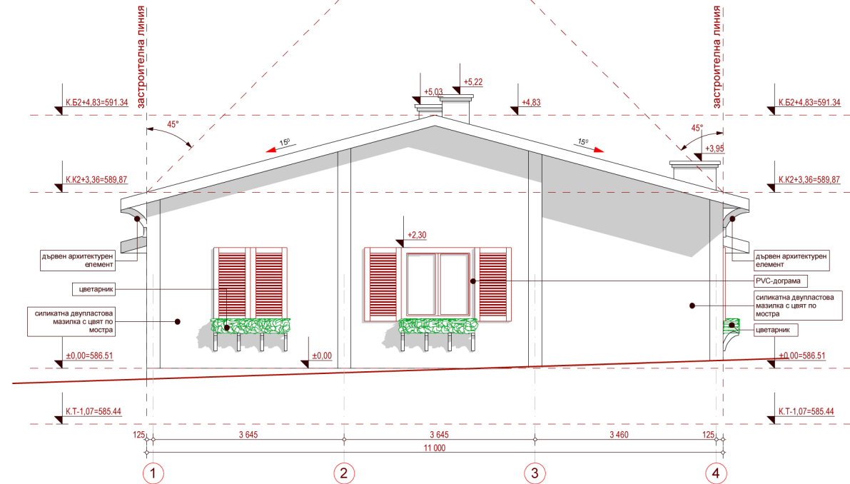
ФАСАДА ЮГ М 1:50
