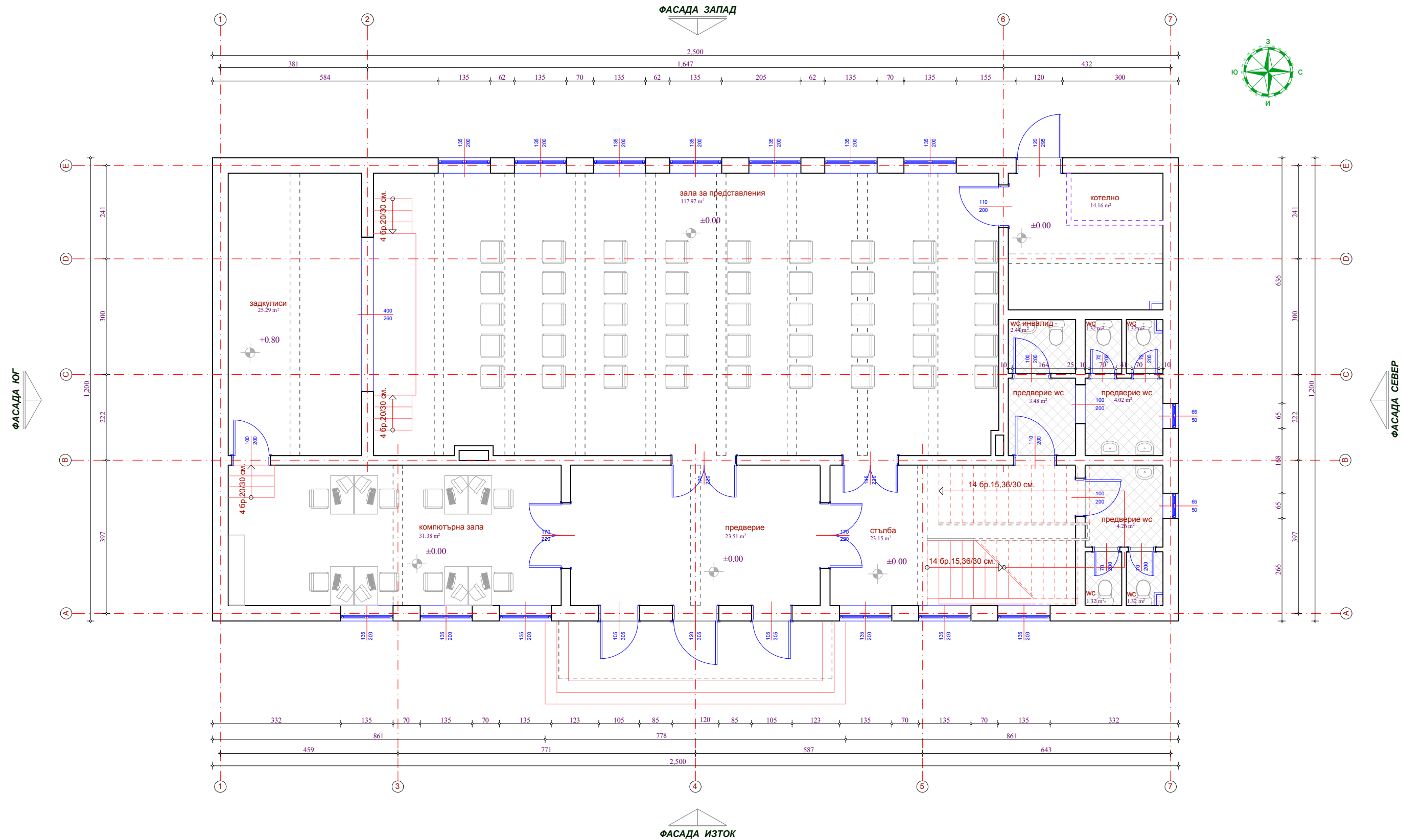
Разпределение I етаж
